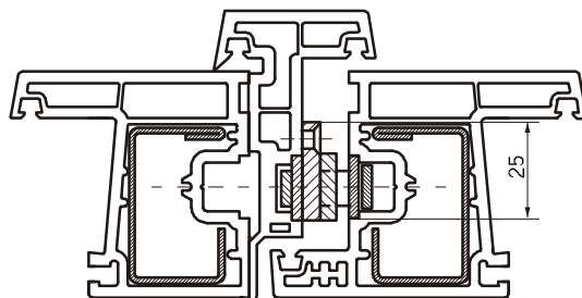
Położenie zatrzasku balkonowego BK WSK 121 na profilu
