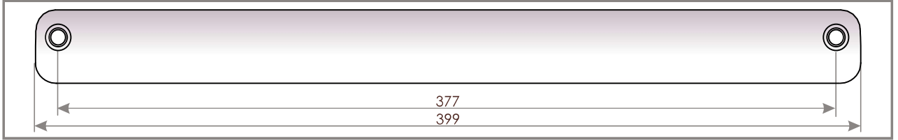
OKAP AKUSTYCZNY OZ 400
