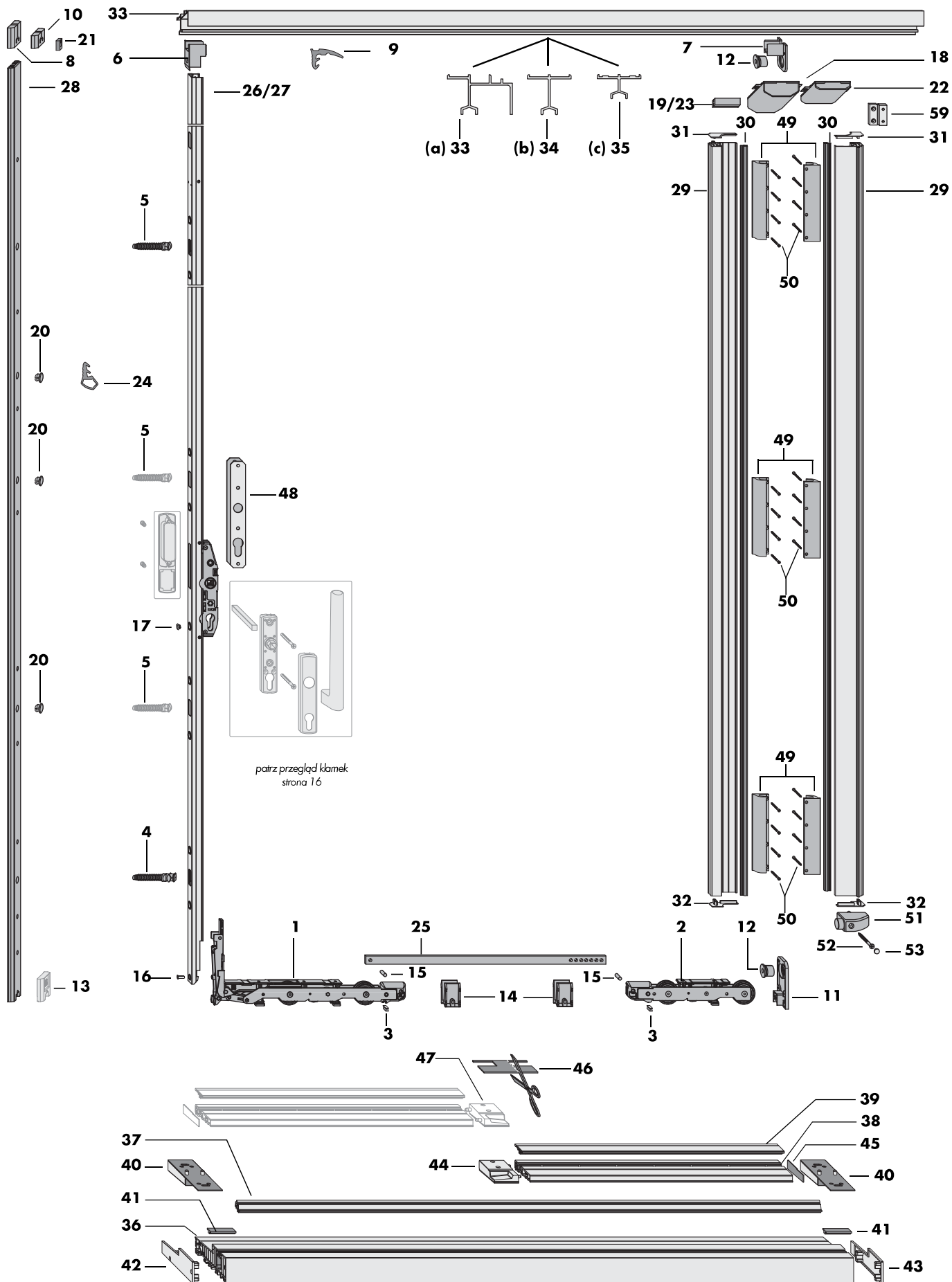
Rys. 1: Rysunek okuć HS 300 schemat A
